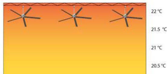
CON L'USO DEI DESTRATIFICATORI
